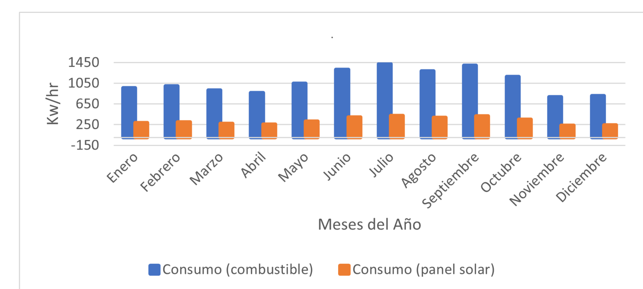
Figura 2 Consumo de combustible vs. placas solares en residencia de 1,700 ft²
