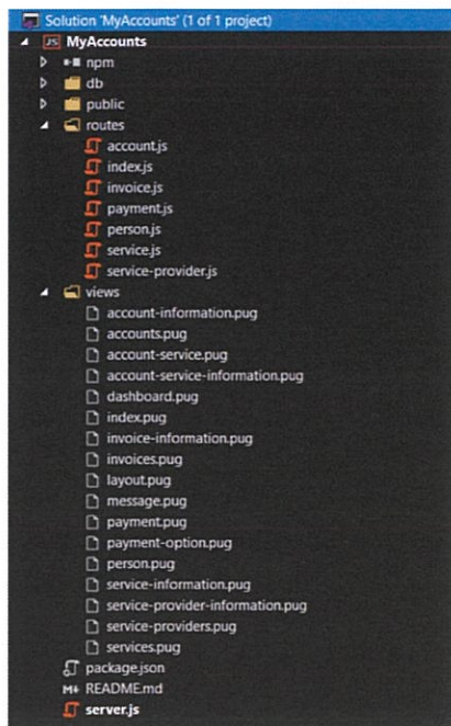
Figure 2 - Estructura de la aplicación web, parte I
