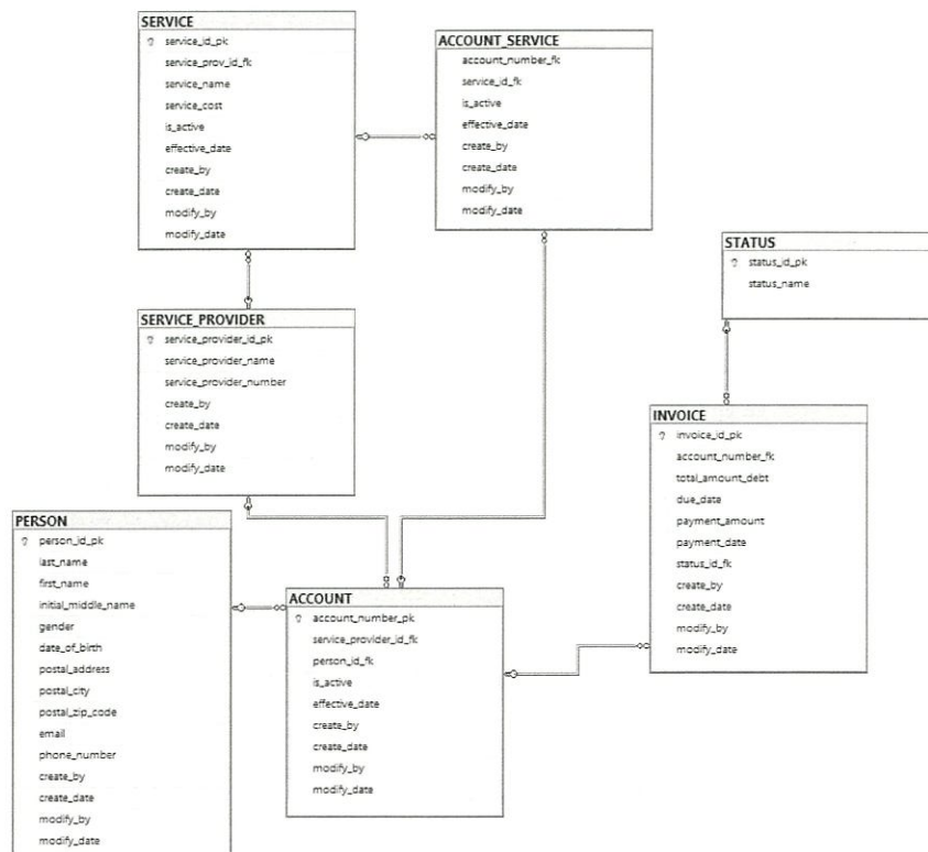
Figure 4 - Diagrama de Entidad Relacional de la Base de Datos
