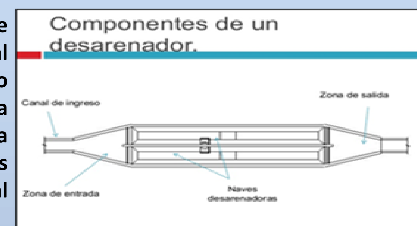
Figura 1 Desarenador flujo horizontal (vista de arriba) [3]
