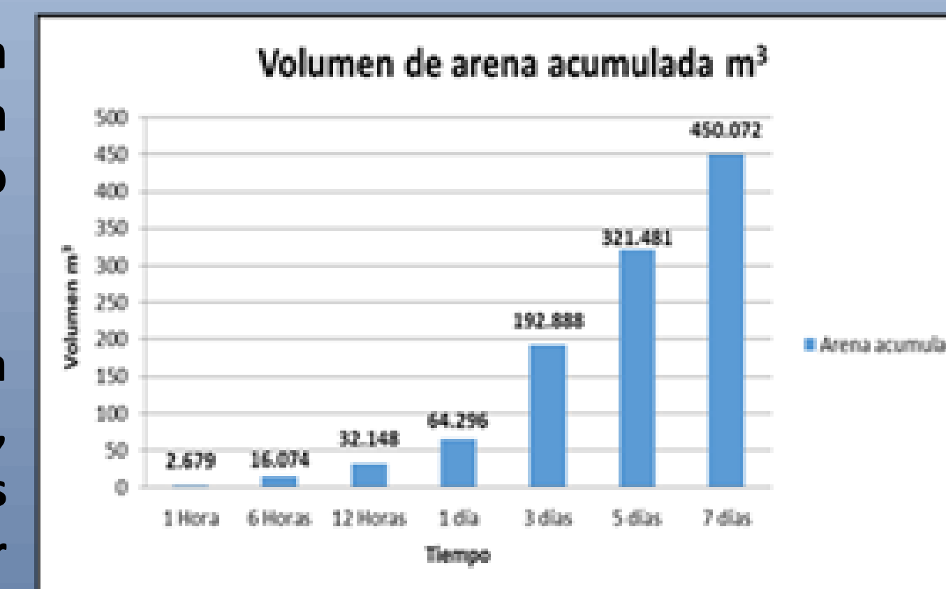
Figura 2 Acumulación de arena [4]
